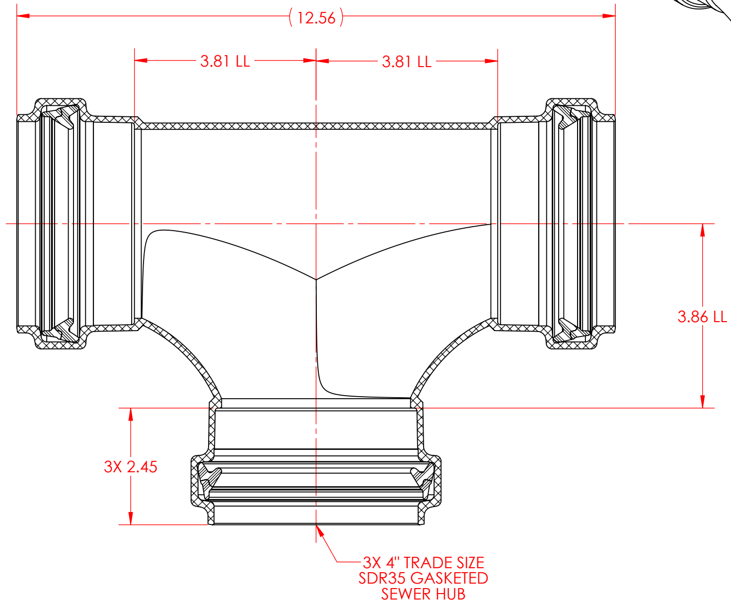
SECTION A-A
