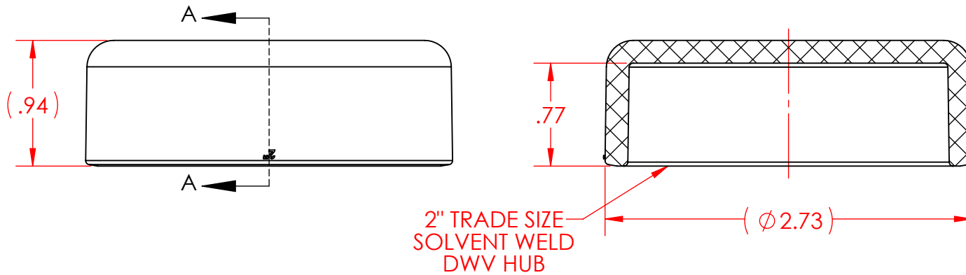
SECTION A-A
