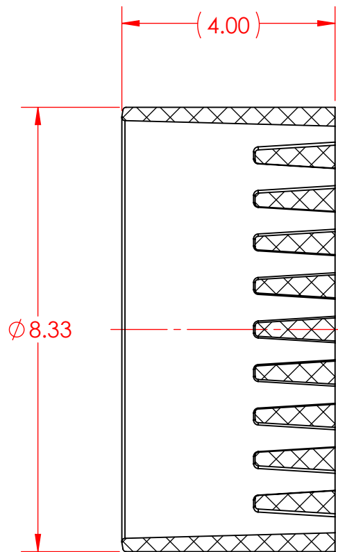
SECTION A-A
