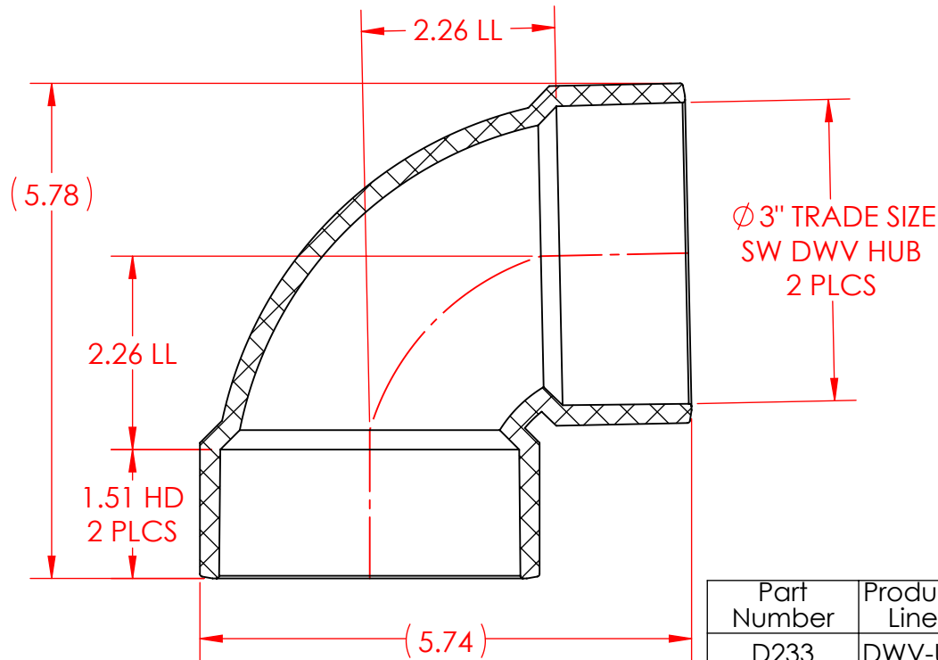
SECTION A-A
