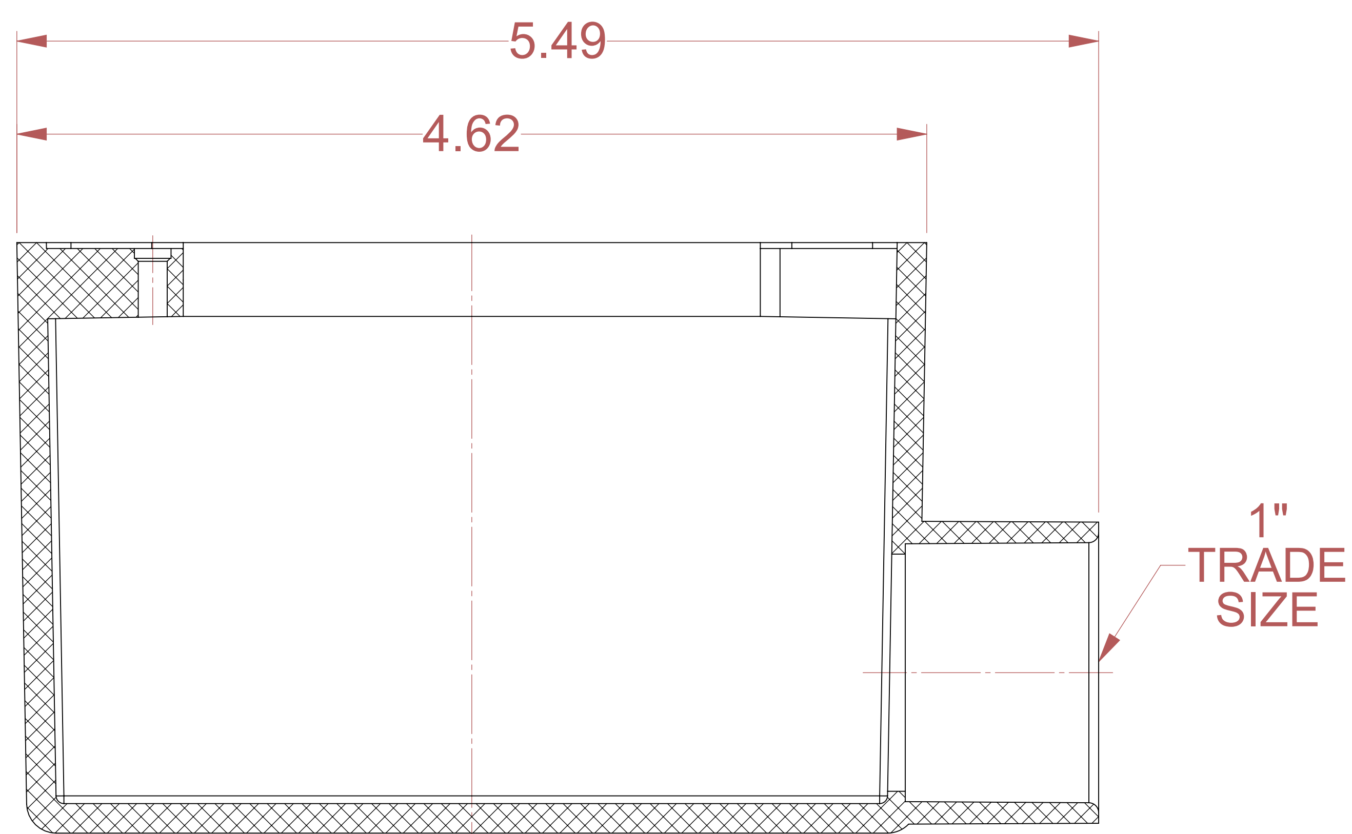
SECTION A-A
