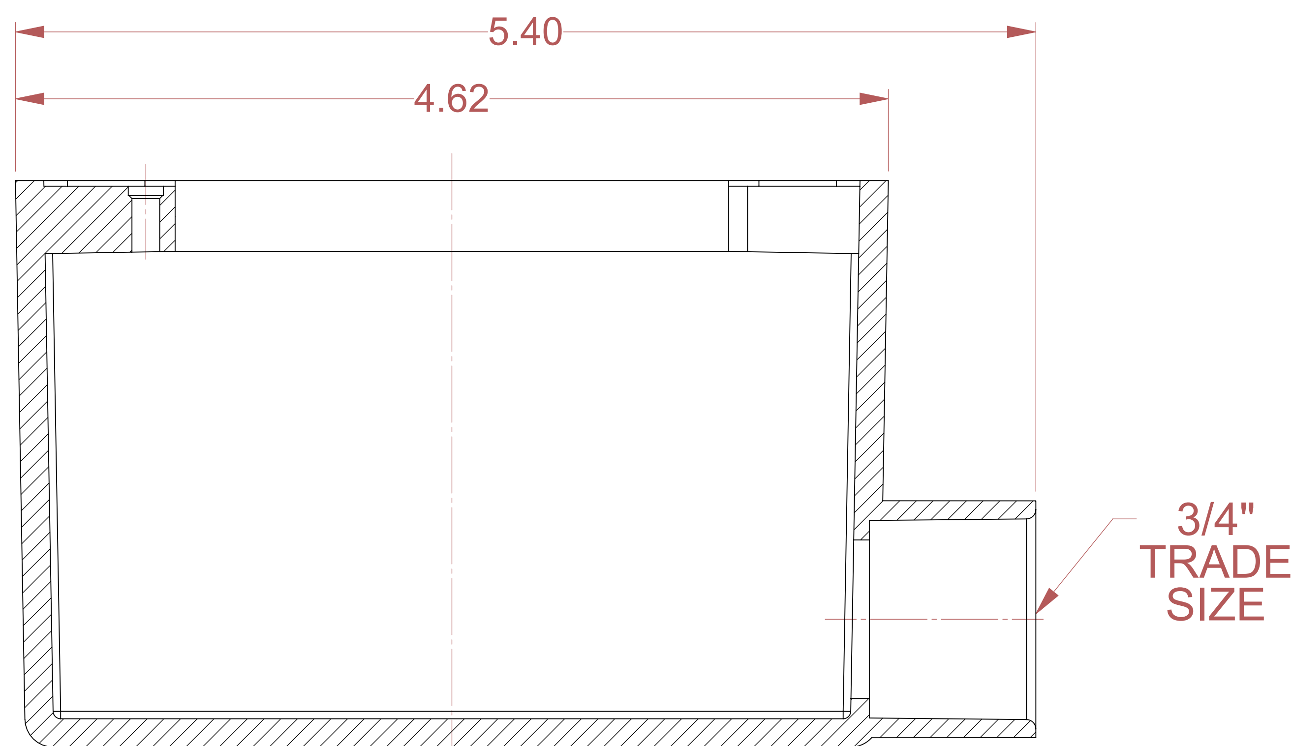
SECTION A-A
