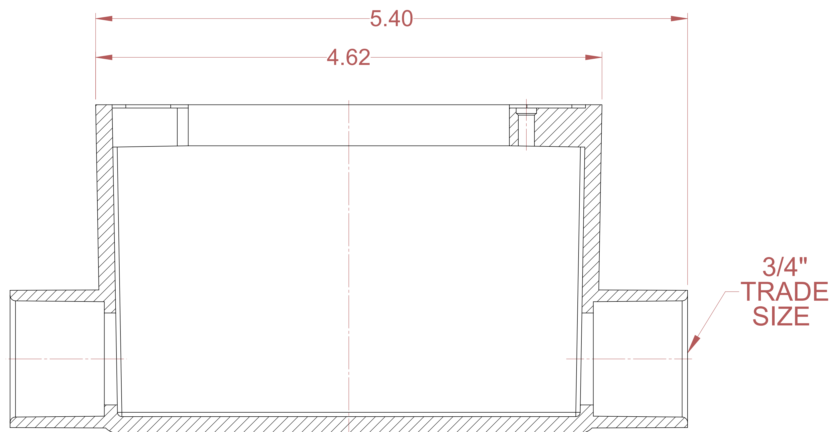
SECTION A-A
